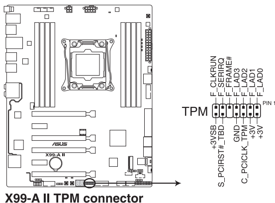
X99-A II TPM connector
