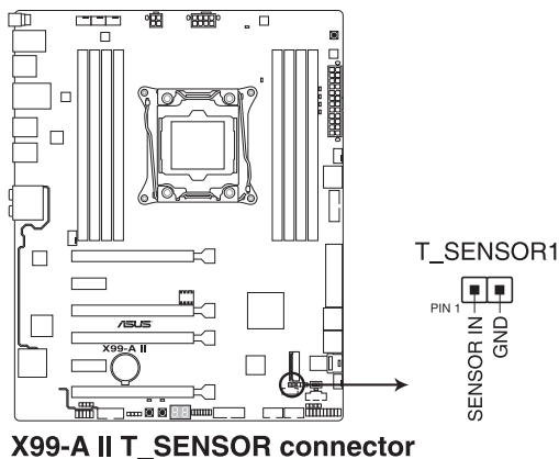
X99-A II T_SENSOR connector
