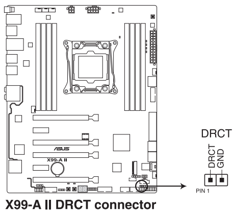
X99-A II DRCT connector
